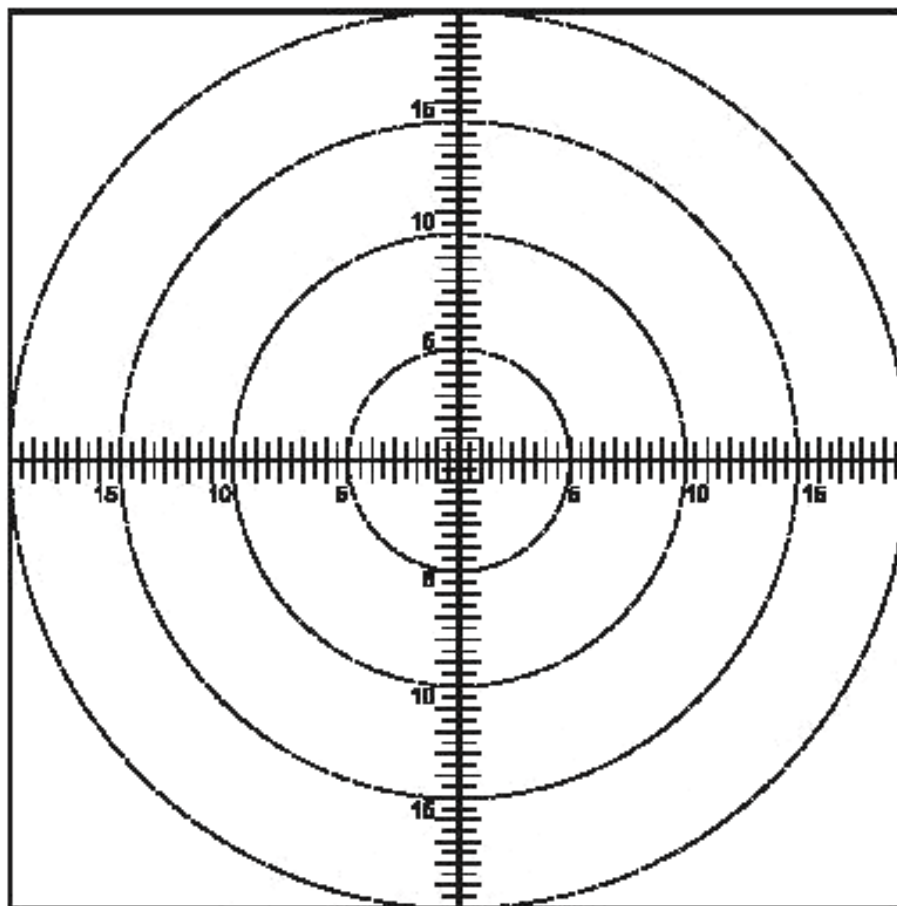
Рисунок 1 — ТЕСТ-ОБЪЕКТ для определения ДИСТОРСИИ ИЗОБРАЖЕНИЯ
