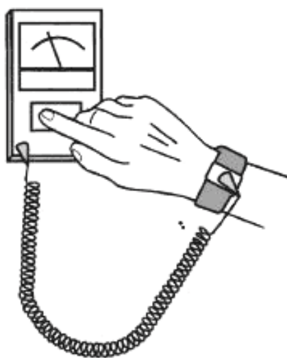
Рисунок А.1 — Испытание антистатического браслета
