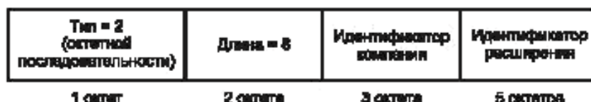
Рисунок 9 — Формат глобального идентификатора в IAS
