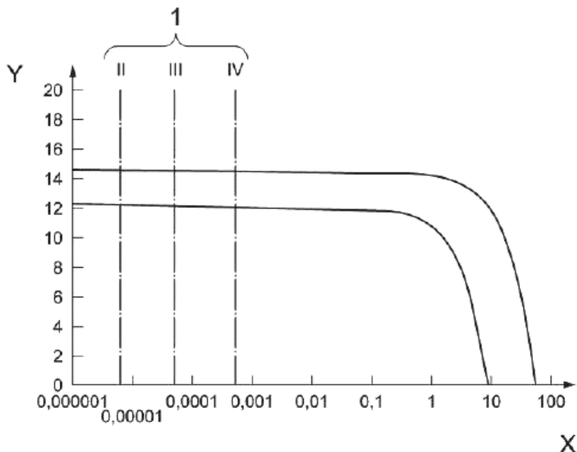
Кривые зрительного представления, позитивная и негативная X – область экрана, занятая дефектами, в процентах от площади; Y – быстрота поиска, символ/с; а – кривая зрительного представления, черный или белый фон (позитивная полярность); б – кривая зрительного представления, белый текст на черном фоне (негативная полярность); 1 – классификация дефектов по ИСО 13406-2,
