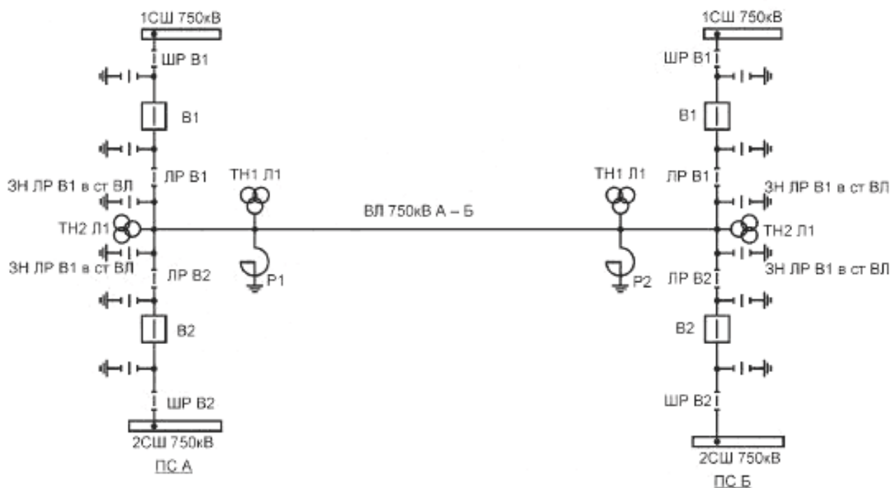
Рисунок Г.2 — Схема подключения ВЛ 750 кВ А-Б
