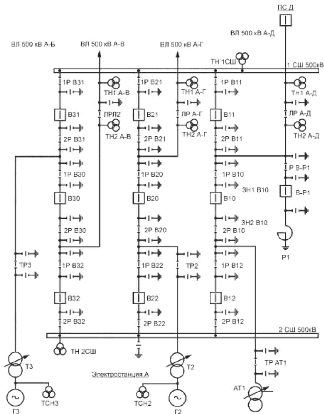
Рисунок Е.4 — Полуторная схема РУ
