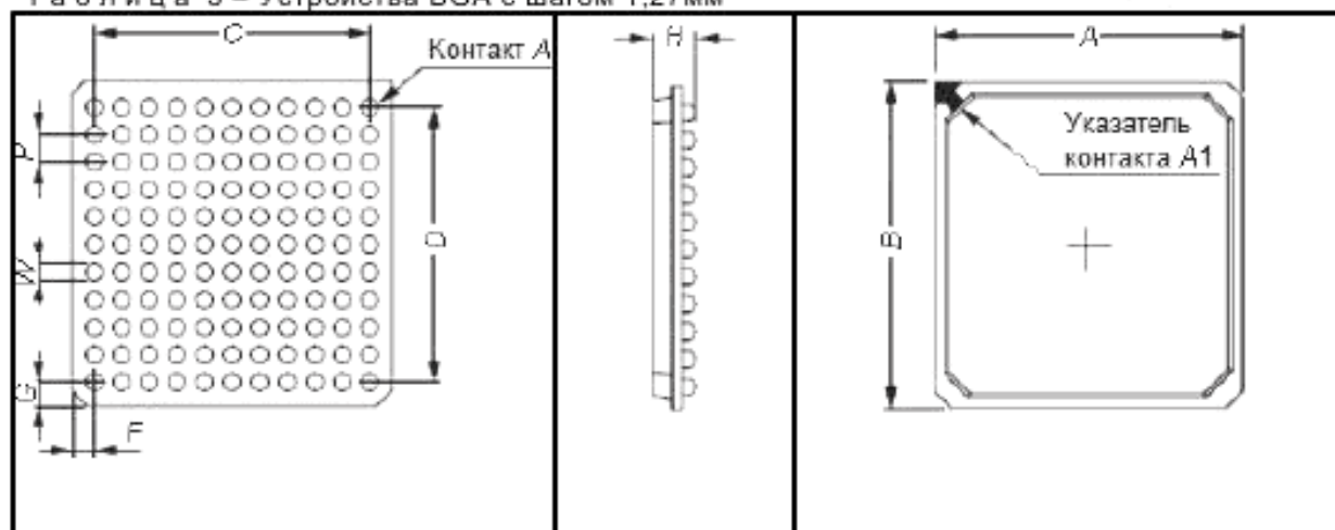
Т а б л и ц а 3 – Устройства BGA с шагом 1,27мм
